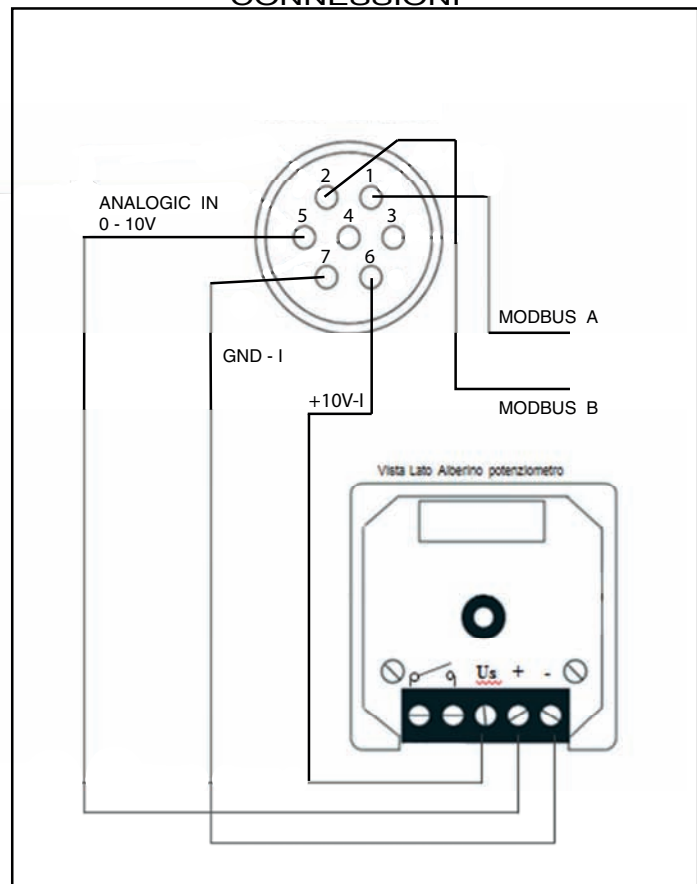
DETTAGLIO CONNESSIONI
