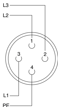
CONNETTORE ALIMENTAZIONE SUPPLY CONNECTOR
