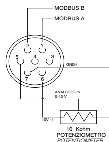
DETTAGLIO CONNESSIONI
