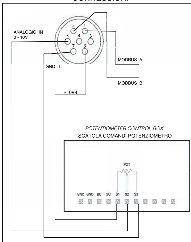
DETTAGLIO CONNESSIONI
